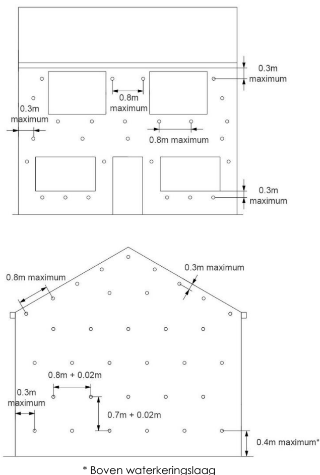
Figuur 1 : Vulpatroon in geval van inblaasmondjes van 18 mm
