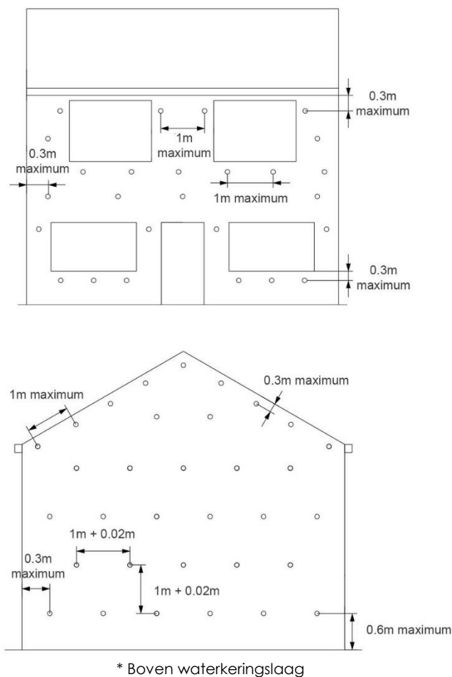
Figuur 2 : Vulpatroon in geval van inblaasmond van 20 mm
